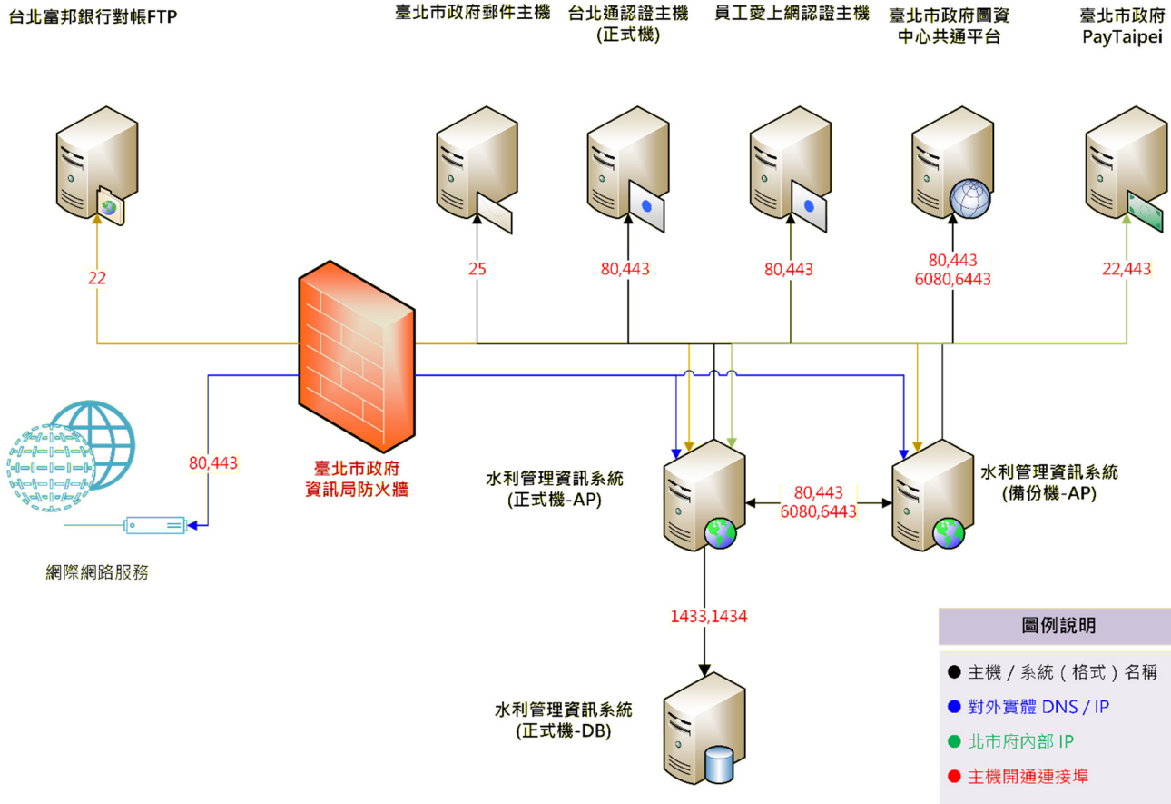
圖 1：硬體架構圖
